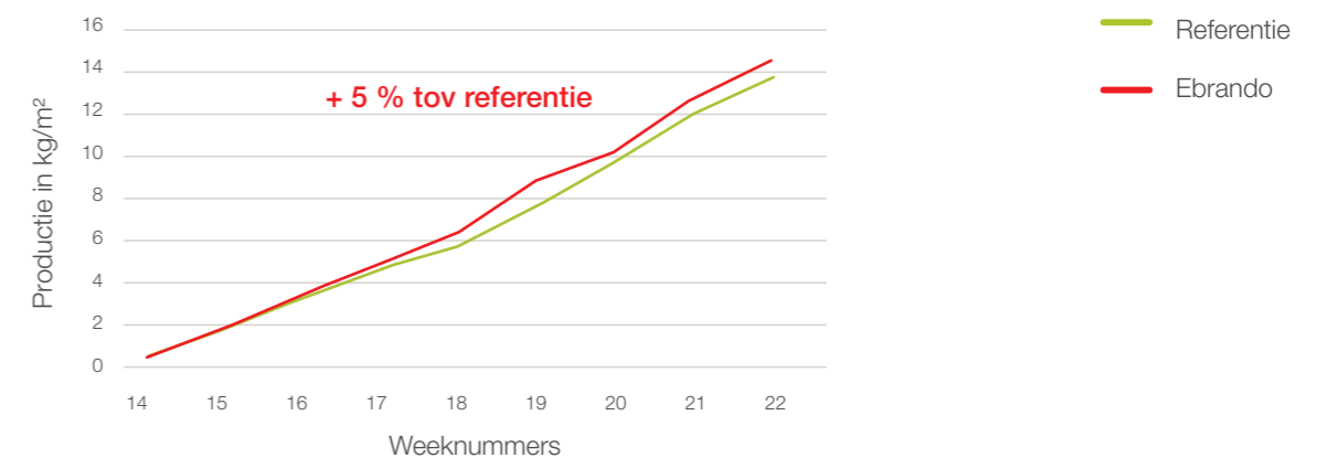
Grafiek 2 - Vroege productie PSKW 2016
