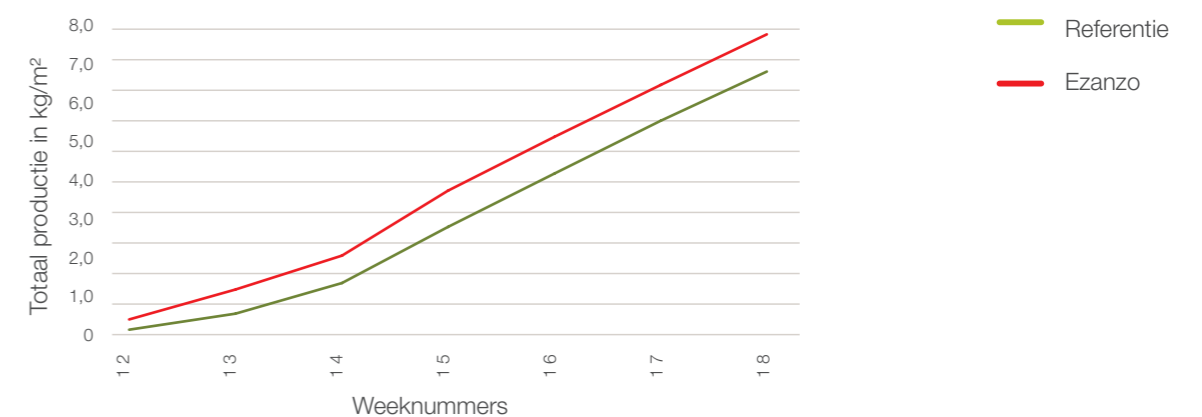
Grafiek 5 - PCH 2018- eerste 6 productieweken
