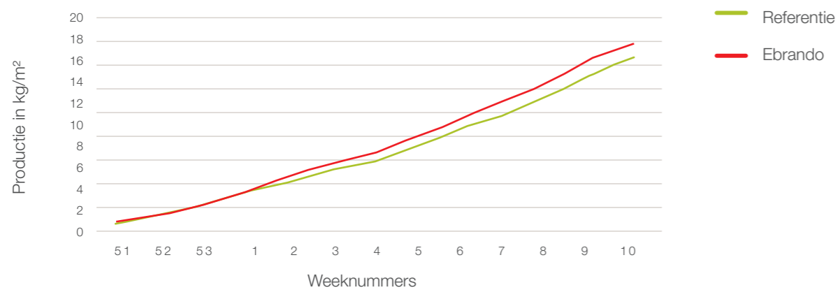
Grafiek 1 - Productieverloop vroege productie belichte teelt 2015-2016 PSKW
