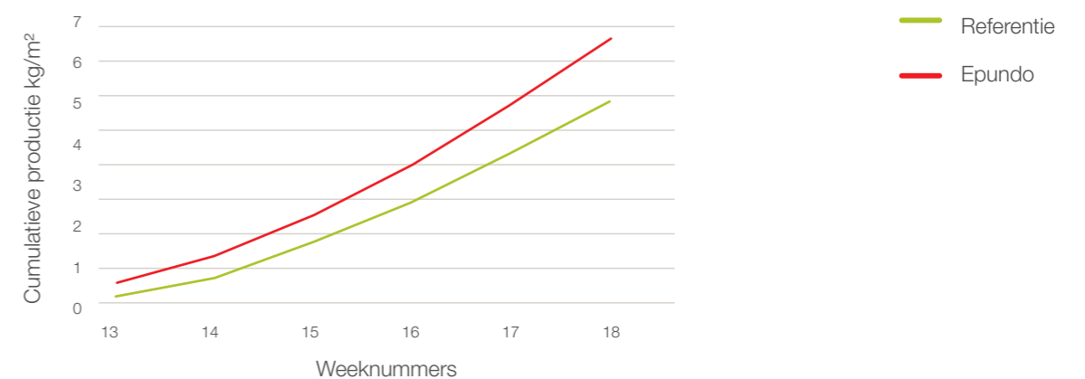
Grafiek 3 - Vroege productie 2017 PCH
