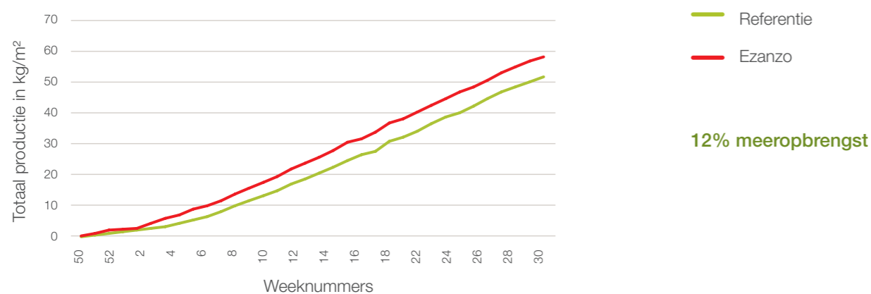
Grafiek 4 - Productieverloop PSKW belichte teelt 2017-2018
